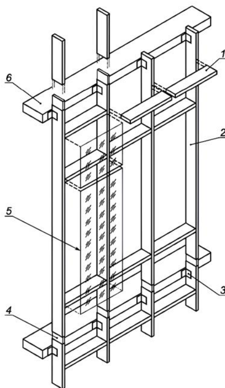
Схема устройства стойечно-ригельной фасадной системы
