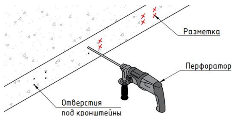
Схема устройства отверстий (Схема показана условно)
