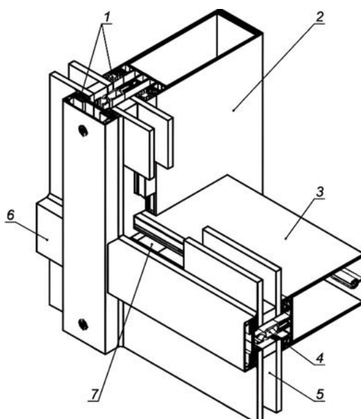
Схема устройства стоечно-ригельной системы с рамным остеклением
