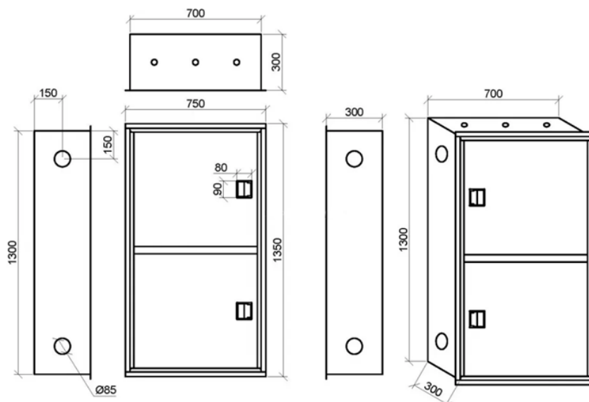
Схема ШП-К-320-12НЗБ
