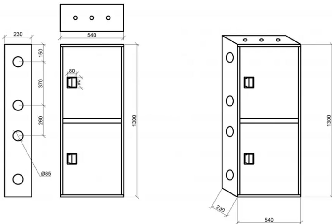
Схема пожарного шкафа ШПК-320 НЗК
