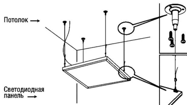
Крепление подвесного светодиодного светильника в подвесном потолке
