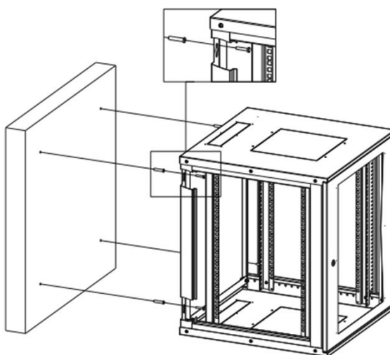
Возможный вариант крепления телекоммуникационного шкафа к стене
