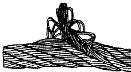
Рисунок 11. Выдавливание сердечника.
